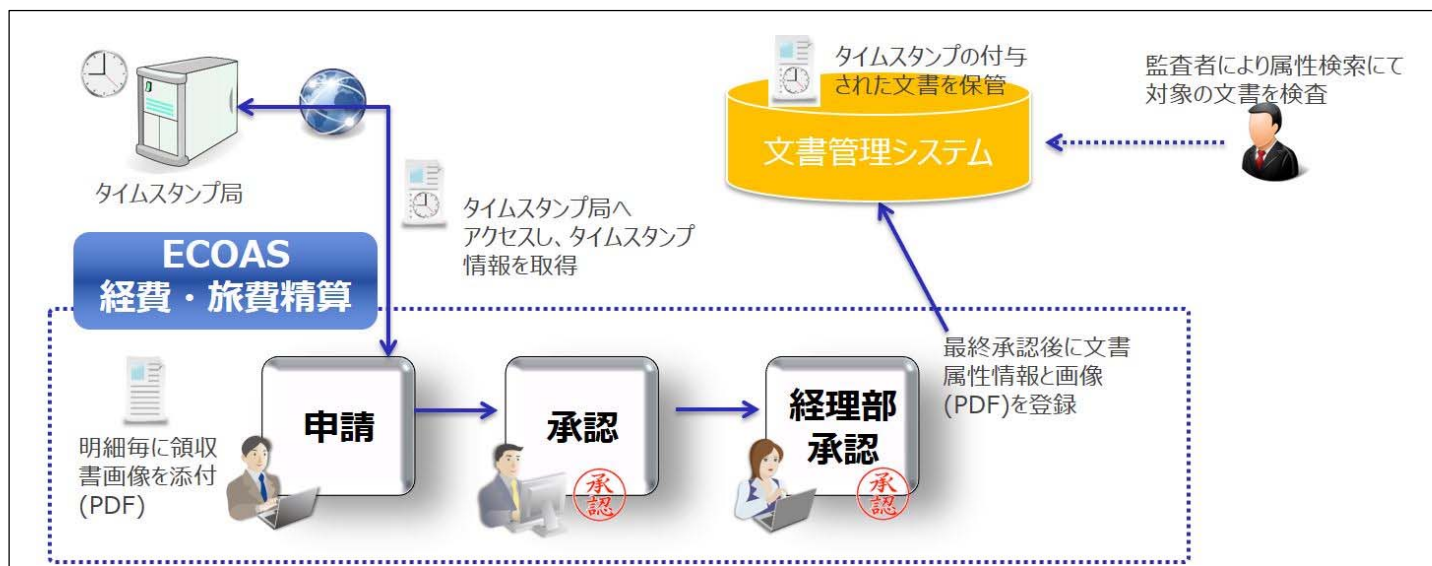
▲「ECOAS 経費・旅費精算」を利用した電子帳簿保存法対応のイメージ図
